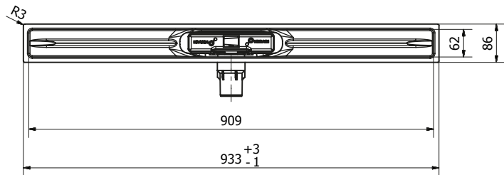
PRO 72 Linear Drain 900mm
